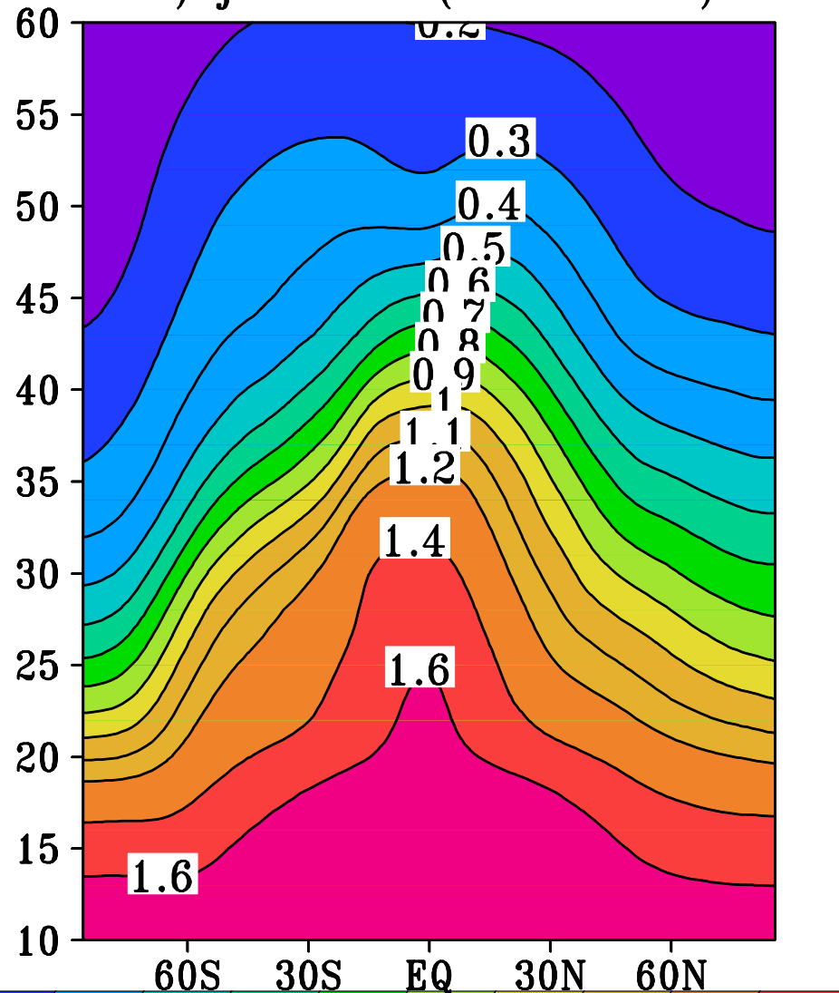
B) xjcin CH 4 (2010–2011)
