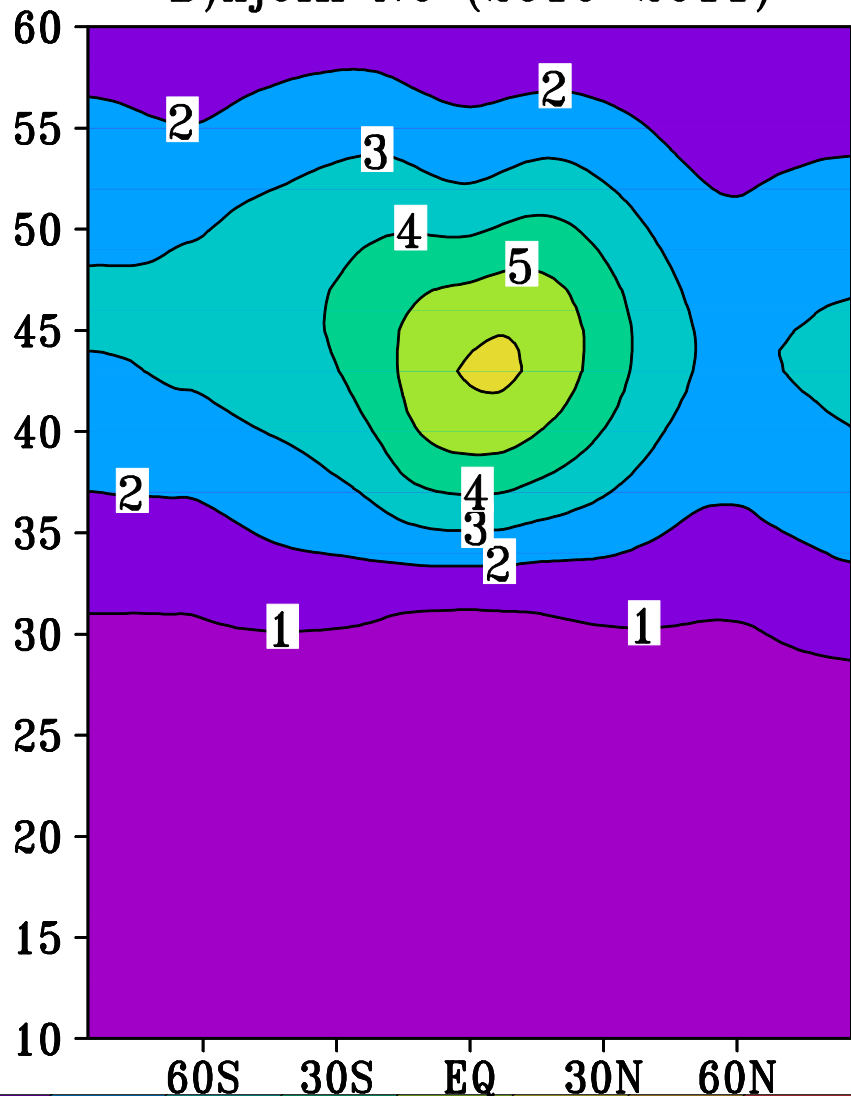
B) xjcin NO (2010–2011)
