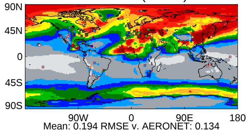
akwxs Total AOD (440nm) MAM
